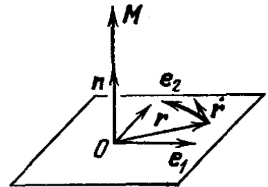
Рис. 28. Кинетический момент
