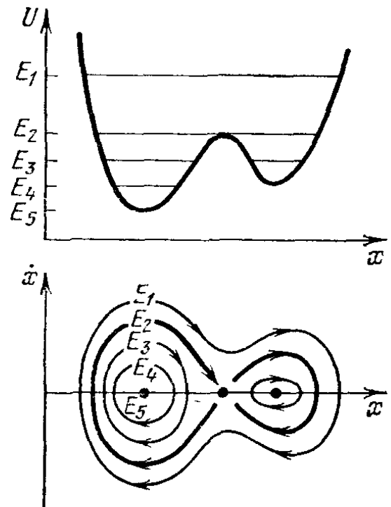
Рис. 10. Потенциальная энергия и фазовые кривые
