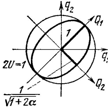
Рис. 80. Конфигурационное пространство связанных маятников
