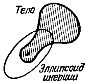
Рис. 116. Эллипсоид инерции
