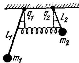
Рис. 84. Связанные маятники
