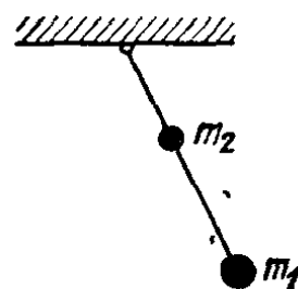
Рис. 87. Предельный случай маятников, связанных бесконечно жесткой пружиной
