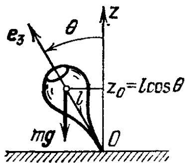
Рис. 125. Волчок Лагранжа
