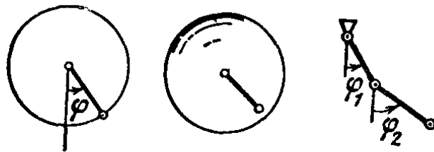
Рис. 58. Плоский, сферический и двойной плоский маятники
