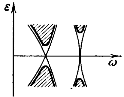
Рис. 100. Влияние трения на параметрический резонанс
