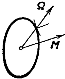
Рис. 119. Угловая скорость, эллипсоид инерции и кинетический момент
