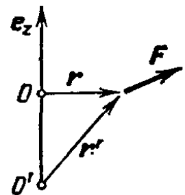
Рис. 37. Момент вектора F относительно оси
