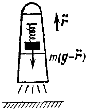
Рис. 107. Перегрузка
