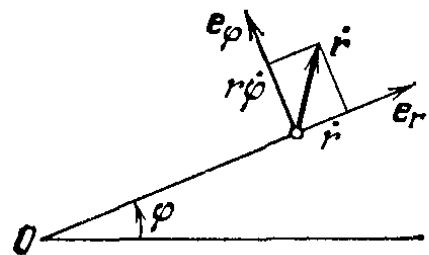
Рис. 29. Разложение вектора \dot{r} по базису e_r, e_\varphi
