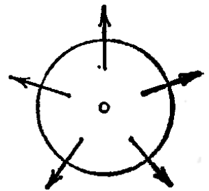
Рис. 163. Поле A
