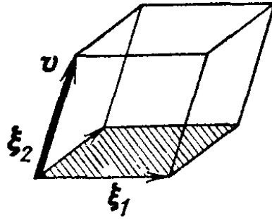
Рис. 137. Поток жидкости через площадку — 2-форма
