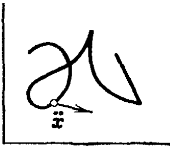
Рис. 3. Траектория движения точки
