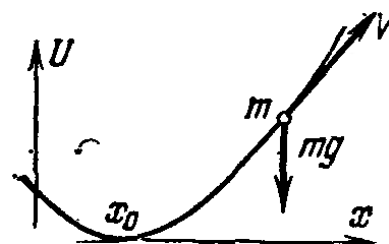
Рис. 77. Бусинка 1 на проволоке
