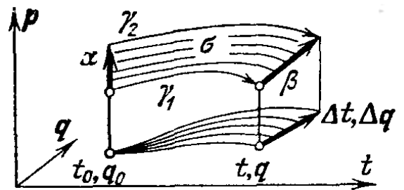
Рис. 200. Вычисление дифференциала функции действия.
