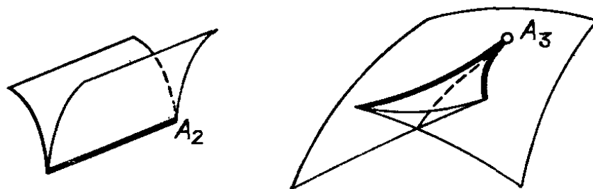
Рис. 256. Типичные особенности волновых фронтов
