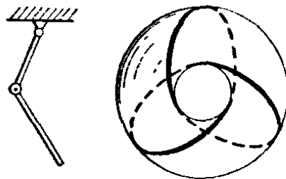
Рис. 191. Периодическое движение двойного маятника
