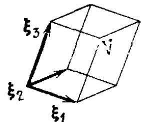
Рис. 138. Ориентированный объем — 3-форма
