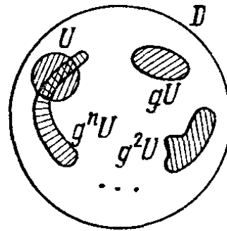
Рис. 51. Теорема о возвращении
