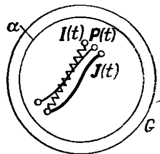
Рис. 226. Доказательство теоремы об усреднении
