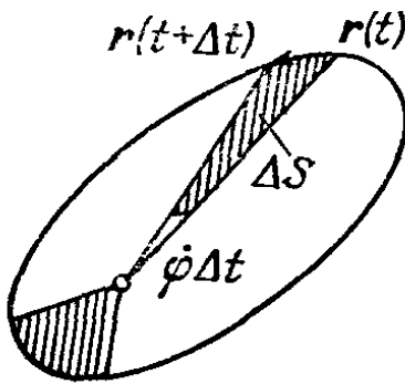
Рис. 30. Секториальная скорость
