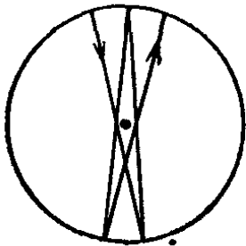
Рис. 111. Траектория маятника Фуко
