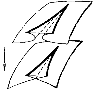
Рис. 263. Раскрытый ласточкин хвост
