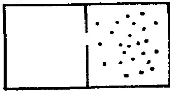
Рис. 50. Молекулы вернулись в первую камеру
