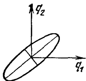
Рис. 85. Потенциальная энергия сильно связанных маятников
