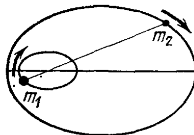
Рис. 40. Задача двух тел
