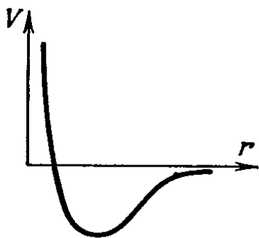
Рис. 34. Эффективный потенциал кеплеровой задачи
