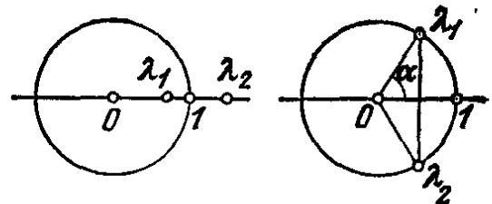
Рис. 97. Собственные числа отображения A
