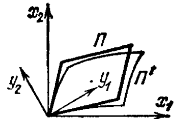
Рис. 159. Независимость внешней производной от системы координат
