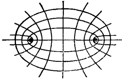
Рис. 205. Конфокальные эллипсы и гиперболы
