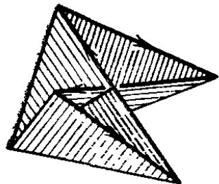
Рис. 164. Конус над циклом
