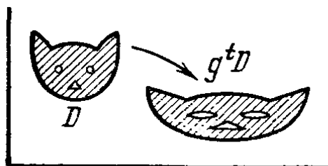
Рис. 48. Сохранение объема
