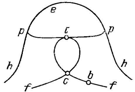
Рис. 259. Классификация точек на поверхности
