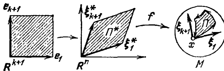
Рис. 156. Криволинейный параллелепипед \Pi
