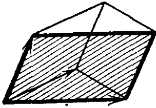
Рис. 136. Ориентированная площадь — 2-форма
