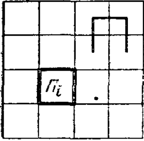
Рис. 160. Доказательство формулы Стокса для параллелепипеда
