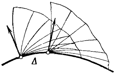
Рис. 233. Параллельное перенесение в пространстве
