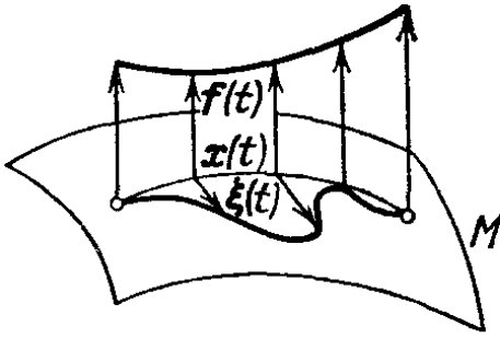
Рис. 72. Лемма о нормальном поле
