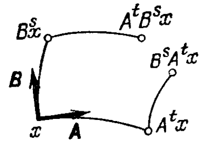
Рис. 169. Некоммутирующие потоки
