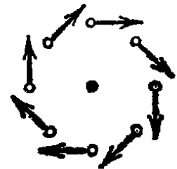
Рис. 27. Непотенциальное поле
