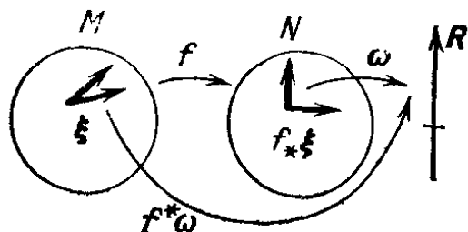
Рис. 149. Форма на N индуцирует форму на M
