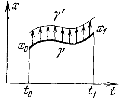
Рис. 41. Вариации кривой
