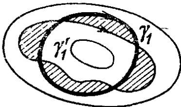
Рис. 218. Независимость переменной действия от выбора кривой интегрирования
