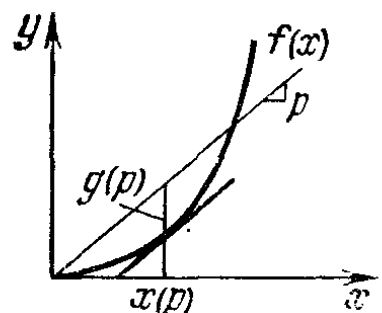
Рис. 43. Преобразование Лежандра
