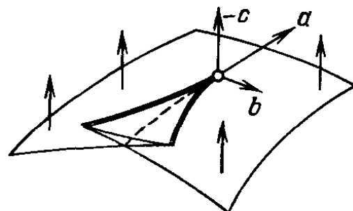
Рис. 257. Векторное поле вблизи ласточкиного хвоста
