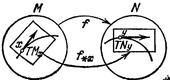
Рис. 64. Производная отображения
