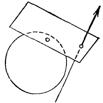
Рис. 253. Пространство ориентированных прямых
