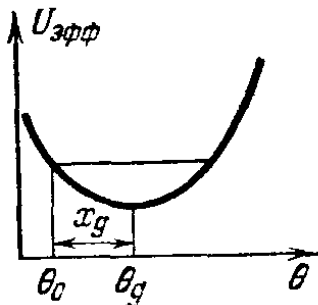
Рис. 133. Определение амплитуды нутации
