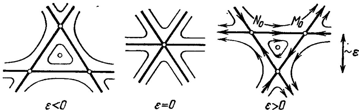
Рис. 239. Прохождение резонанса 3 : 1
