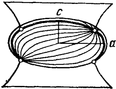
Рис. 207. Геодезические, выходящие из точек округления
