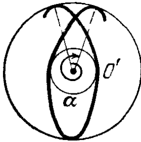
Рис. 123. Траектория точки касания на неподвижной плоскости
