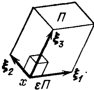
Рис. 155. К определению дивергенции векторного поля
