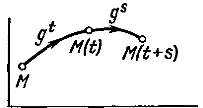
Рис. 14. Фазовый поток
