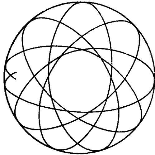
Рис. 33. Всюду плотная в кольце орбита
