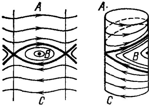
Рис. 220. Переменные действие — угол на симплектическом многообразии
