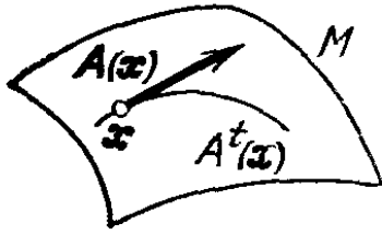
Рис. 168. Группа диффеоморфизмов, заданная векторным полем
