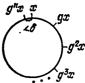
Рис. 52. Всюду плотное множество на окружности
