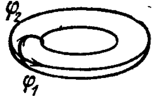
Рис. 53. Тор
