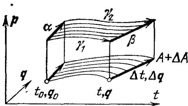
Рис. 202. Функция действия как решение уравнения Гамильтона — Якоби
