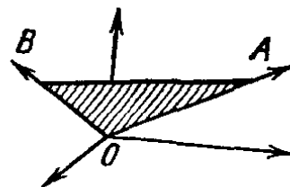
Рис. 60. Конфигурационное пространство треугольника
