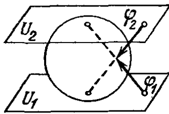
Рис. 57. Атлас сферы
