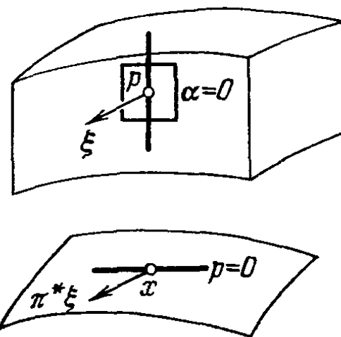
Рис. 237. Симплектизация контактного многообразия
