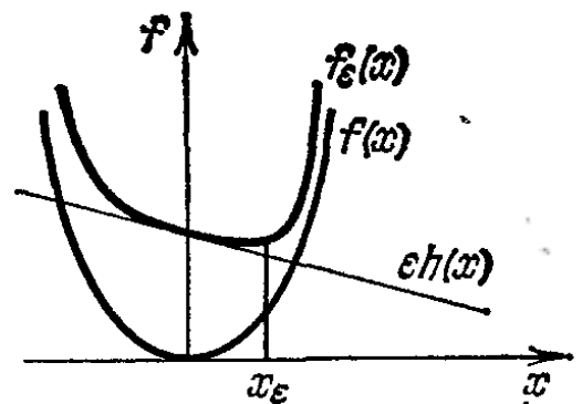
Рис. 132. Перемещение минимума при малом изменении функции
