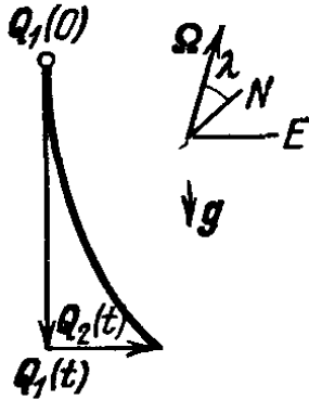
Рис. 109. Отклонение падающего камня силой Кориолиса
