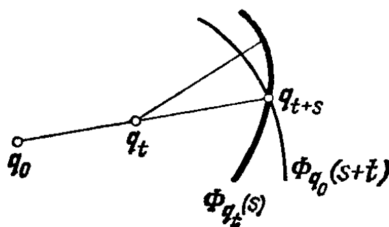
Рис. 194. Доказательство теоремы Гюйгенса
