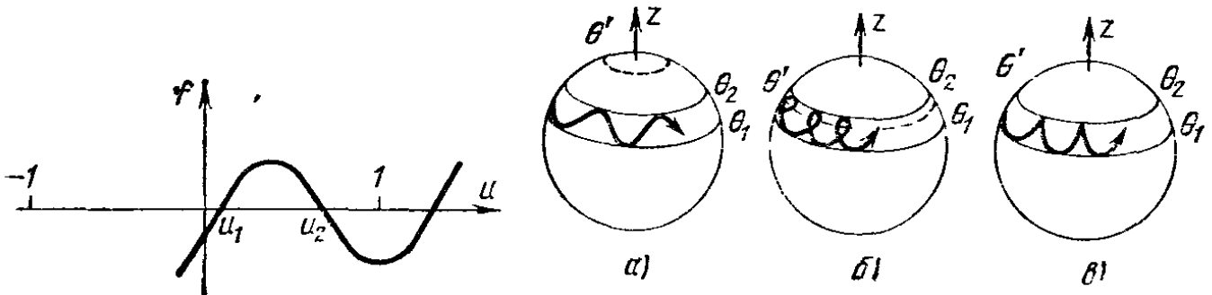
Рис. 127. График функции f(u)
