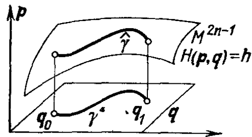
Рис. 189. Принцип Мопертюи
