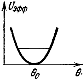
Рис. 130. Эффективная потенциальная энергия волчка
