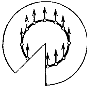
Рис. 231. Параллельное перенесение на сфере
