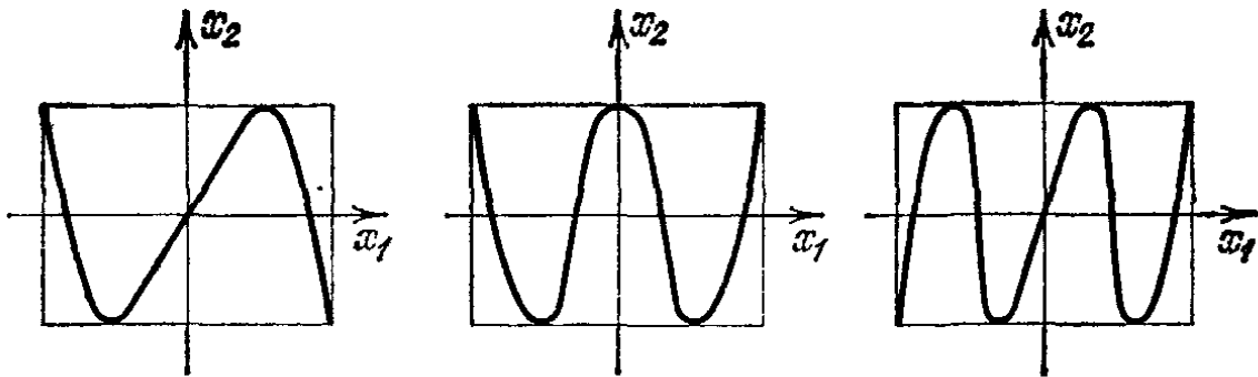
Рис. 24. Многочлены Чебышева
