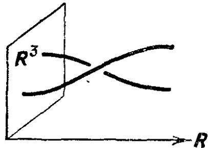
Рис. 4. Мировые линии
