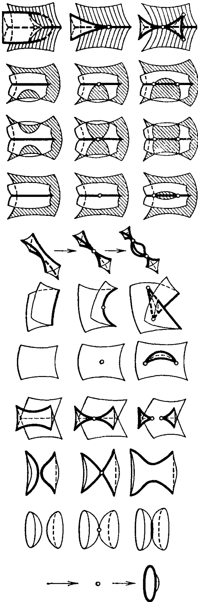
Рис. 255. Типичные перестройки каустики
