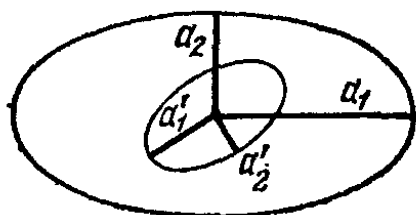
Рис. 90. Полуоси внутреннего эллипсоида меньше
