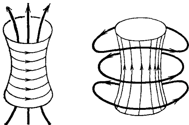
Рис 250. Магнитные поля токов на гиперболоиде
