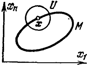
Рис. 61. Вложенное подмногообразие
