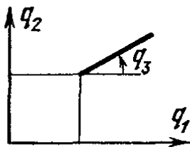
Рис. 59. Конфигурационное пространство отрезка на плоскости
