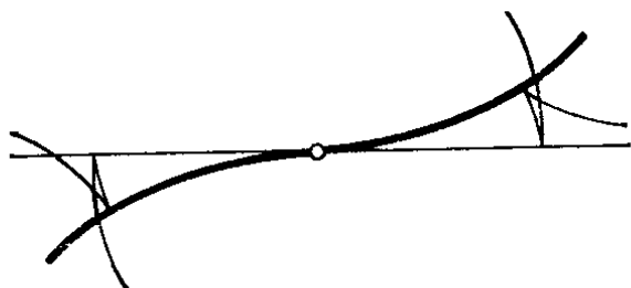
Рис. 264. Эвольвенты кубической параболы
