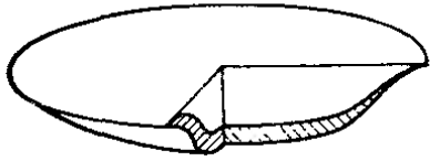
Рис. 254. Новорожденная каустика
