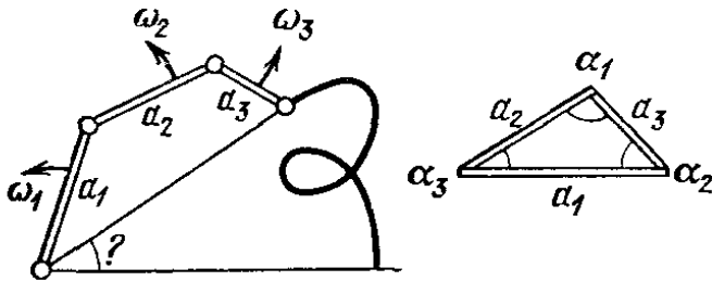
Рис. 223. К задаче о среднем движении перигелиев
