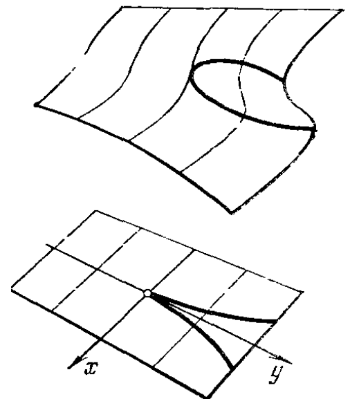
Рис. 245. Сборка Уитни
