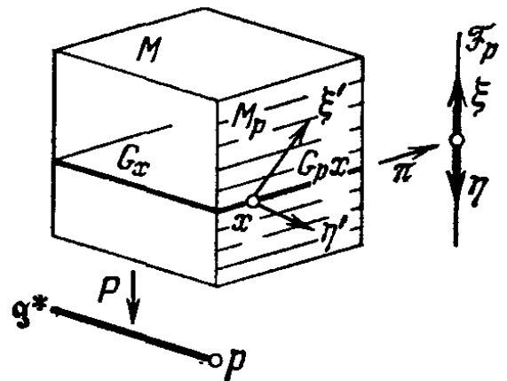
Рис. 238. Приведенное фазовое пространство
