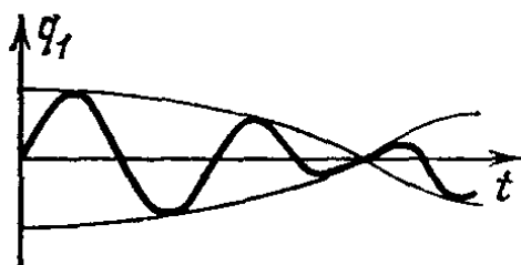
Рис. 83. Биения
