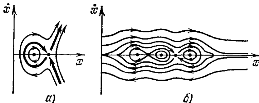
Рис. 12. Фазовые кривые
