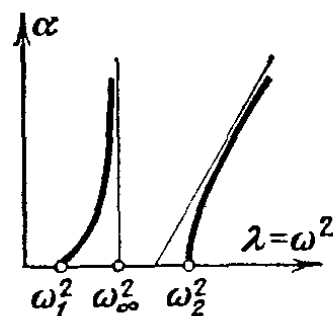
Рис. 86. Зависимость собственных частот от жесткости пружины
