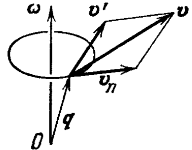
Рис. 106. Сложение скоростей
