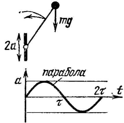
Рис. 102. Перевернутый маятник с колеблющейся точкой подвеса
