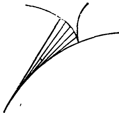
Рис. 252. Особенность эволюенты гладкой кривой
