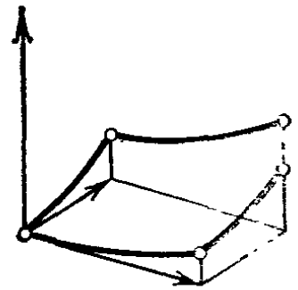
Рис. 236. Интегральные кривые, построенные по неинтегрируемому полю плоскостей
