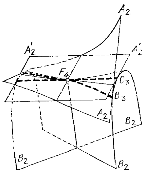
Рис. 266. Фокальные точки поверхности с краем
