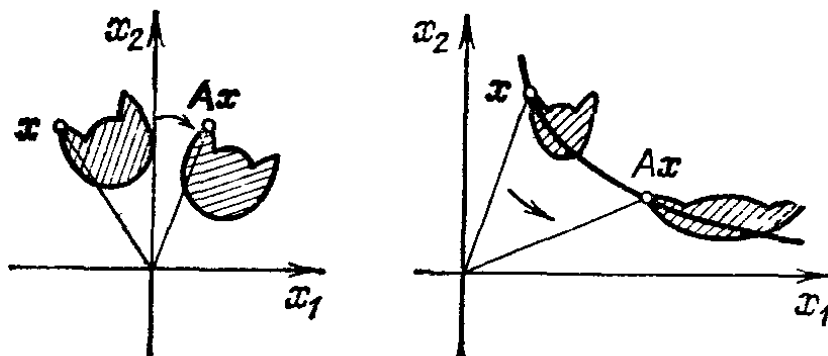
Рис. 96. Поворот и гиперболический поворот
