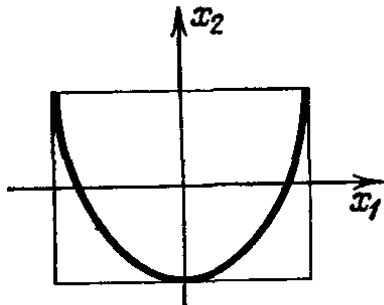
Рис. 22. Фигура Лиссажу с \omega = 2
