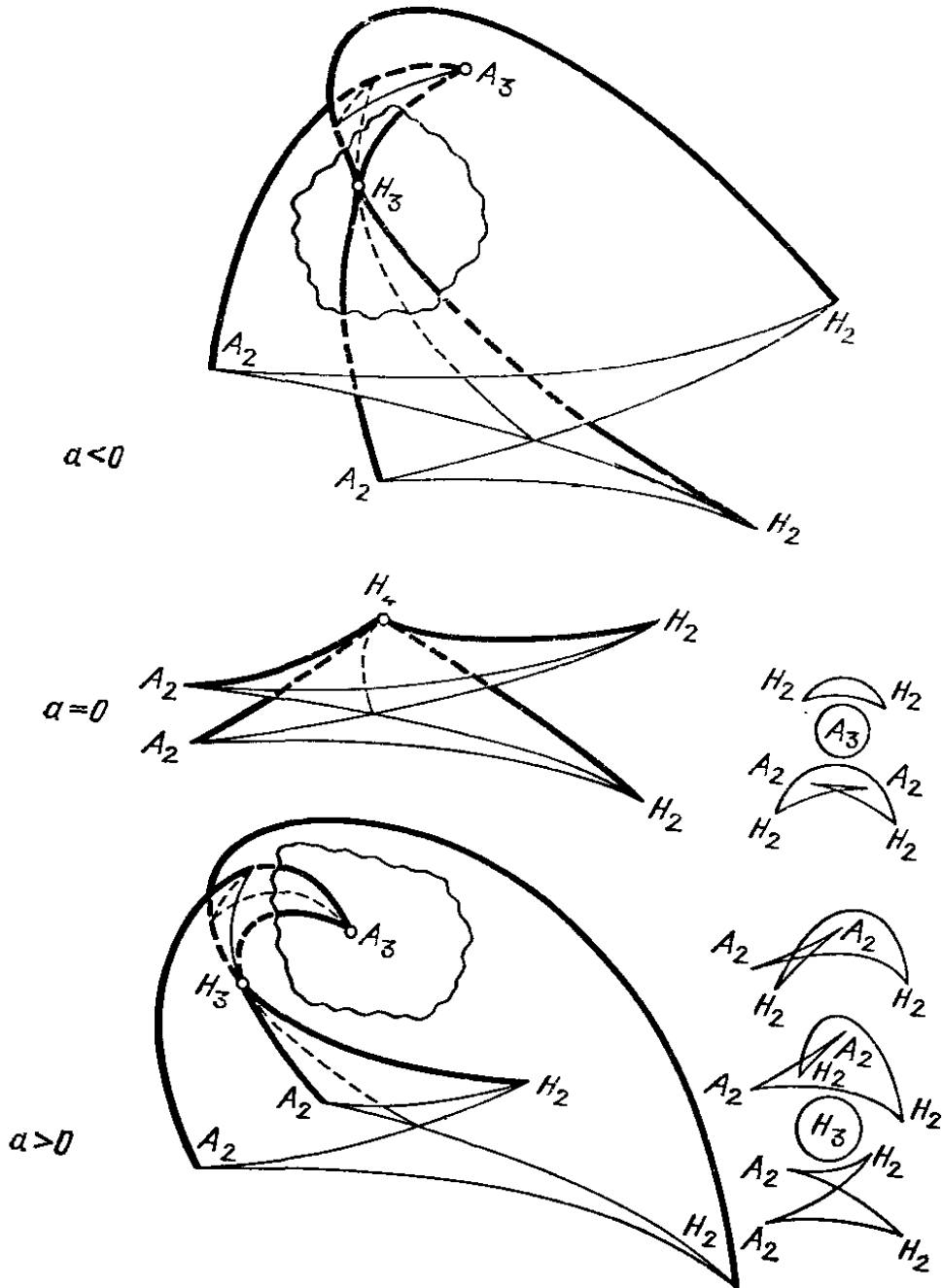
Рис. 269. Типичная перестройка фронта при обходе препятствия
