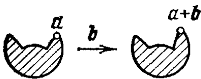
Рис. 1. Параллельный перенос
