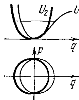
Рис. 76. Линеаризация
