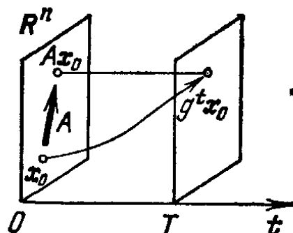
Рис. 95. Отображение на период
