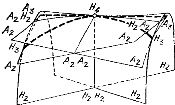
Рис. 268. Каустика группы H_4
