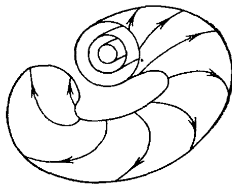
Рис. 242. Инвариантные торы в трехмерном многообразии уровня энергии
