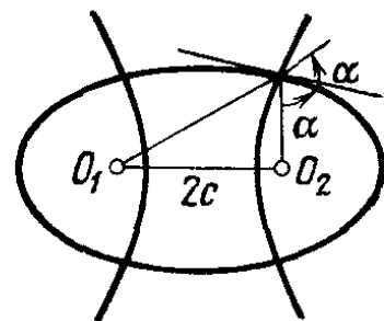
Рис. 204. Эллиптические координаты
