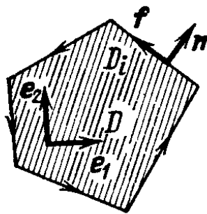
Рис. 152. Ориентация границы
