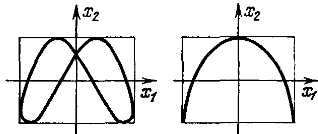
Рис. 23. Серия фигур Лиссажу с \omega = 2
