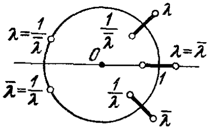
Рис. 176. Расположение собственных чисел симплектического преобразования
