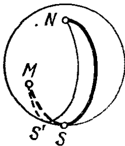
Рис. 190. Неминимальная геодезическая
