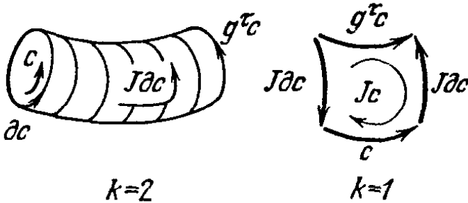
Рис. 167. След цепи при гомотопии
