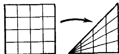
Рис. 162. Доказательство формулы Стокса для симплекса
