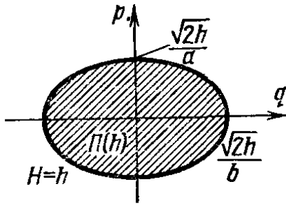
Рис. 217. Переменная действия для гармонического осциллятора
