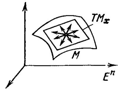
Рис. 62. Касательное пространство
