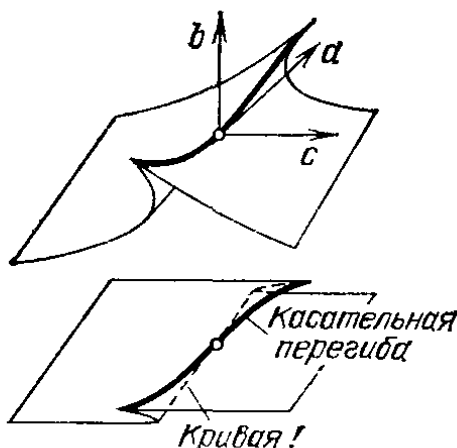
Рис. 265. Поверхность многочленов с кратными корнями
