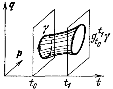
Рис. 183. Интегральный инвариант Пуанкаре
