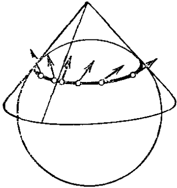
Рис. 231. Параллельное перенесение на сфере
