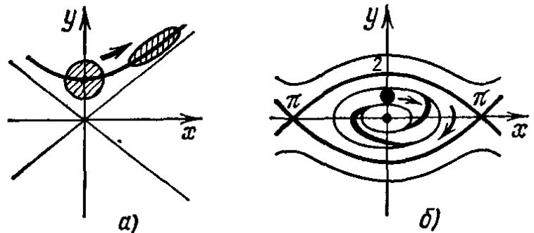
Рис. 15. Действие фазового потока на круг
