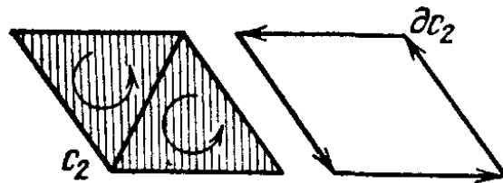
Рис. 153. Граница цепи
