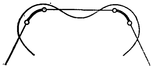
Рис. 262. Кратчайший путь в обход препятствия
