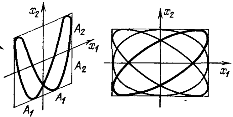
Рис. 20. Серия фигур Лиссажу с \omega = 1
