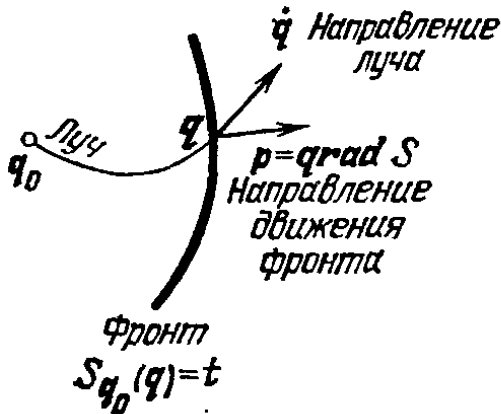
Рис. 195. Направление луча и направление движения фронта
