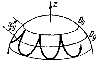
Рис. 134. Движение оси волчка
