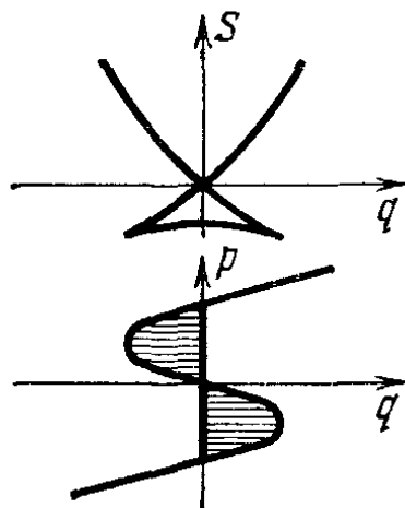
Рис. 203. Типичная особенность решения уравнения Гамильтона — Якоби
