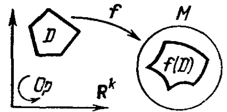
Рис. 150. Сингулярный k -мерный полиэдр
