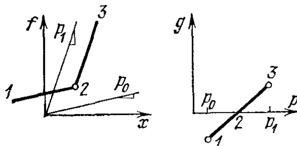
Рис. 44. Преобразование Лежандра переводит угол в отрезок
