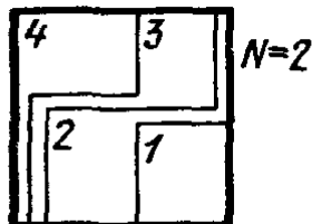
Рис. 172. Переход от одной пары сторон к другой
