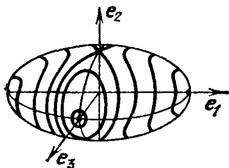
Рис. 121. Траектории уравнений Эйлера на поверхности уровня энергии
