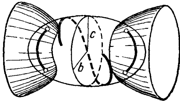
Рис. 208. Геодезические эллипсоида, касающиеся двухполостного гиперboloида
