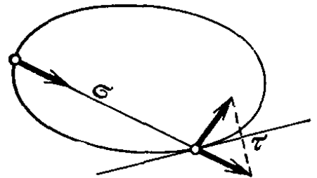
Рис. 261. Бильярдное преобразование как произведение двух инволюций
