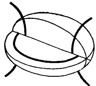
Рис. 249. Фокальный эллипс и фокальная гипербола
