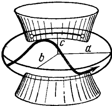
Рис. 206. Геодезическая на трехосном эллипсоиде
