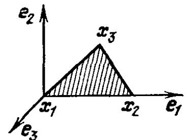
Рис. 112. Конфигурационное многообразие твердого тела
