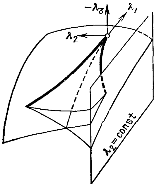
Рис. 247. Пуассонова структура пространства многочленов
