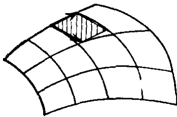
Рис. 147. Интегрирование 2-формы по поверхности
