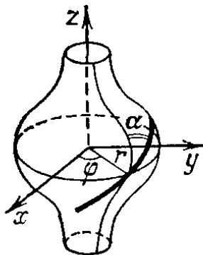
Рис. 66. Поверхность вращения
