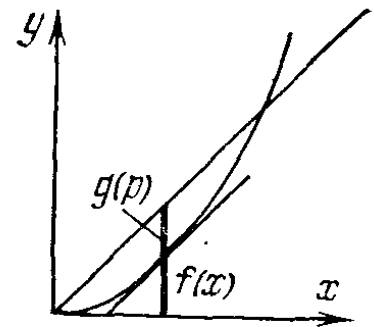
Рис. 46. Преобразование Лежандра квадратичной формы
