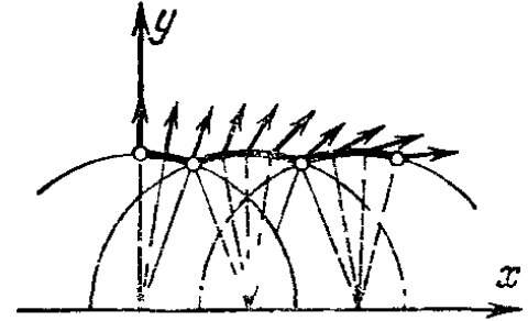
Рис. 232. Параллельное перенесение на плоскости Лобачевского
