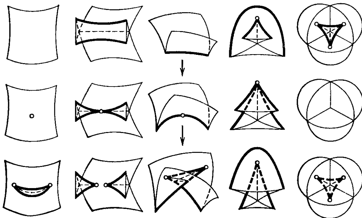
Рис. 258. Типичные перестройки волновых фронтов
