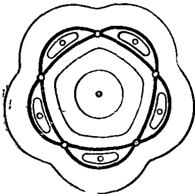
Рис. 241. Усредненный гамильтониан фазовых колебаний вблизи резонанса 5 : 1
