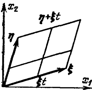
Рис. 158. К теореме о внешней производной
