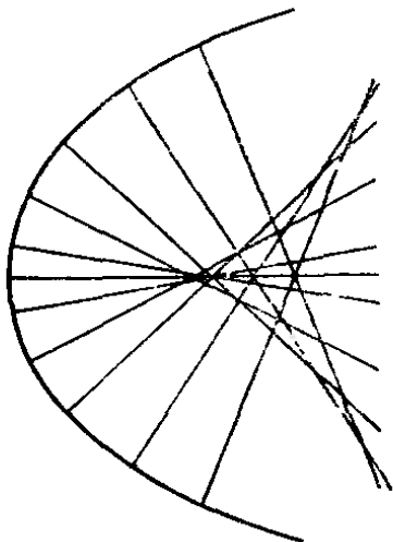
Рис. 251. Система нормалей к параболе
