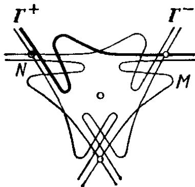
Рис. 240. Расщепление сепаратрис
