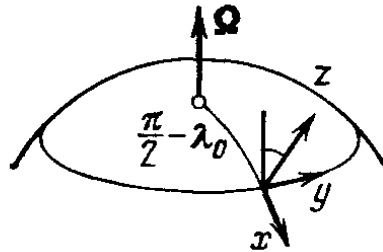
Рис. 110. Система координат для исследования движения маятника Фуко
