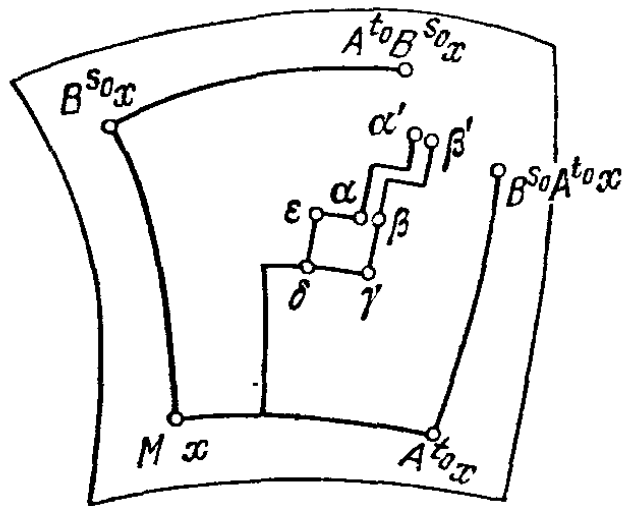
Рис. 171. Криволинейный четырехугольник \alpha\beta\gamma\delta\alpha\beta
