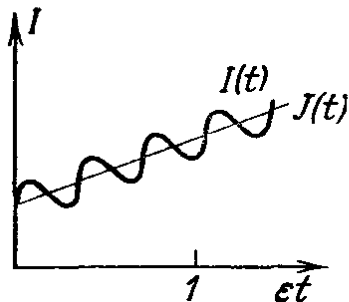
Рис. 224. Эволюция и осцилляции
