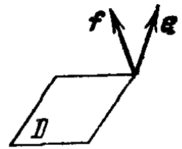
Рис. 174. Косоортogonalное дополнение
