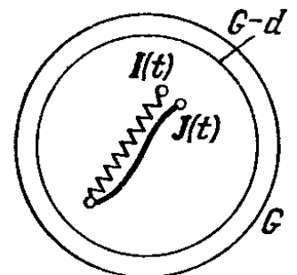
Рис. 225. Теорема об усреднении
