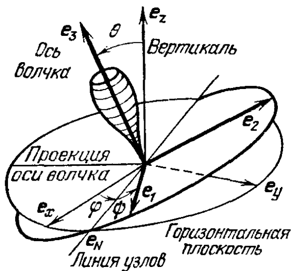
Рис. 126. Углы Эйлера
