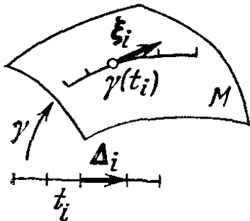
Рис. 146. Интегрирование 1-формы по пути
