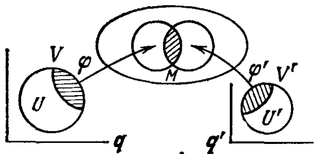
Рис. 56. Совместные карты
