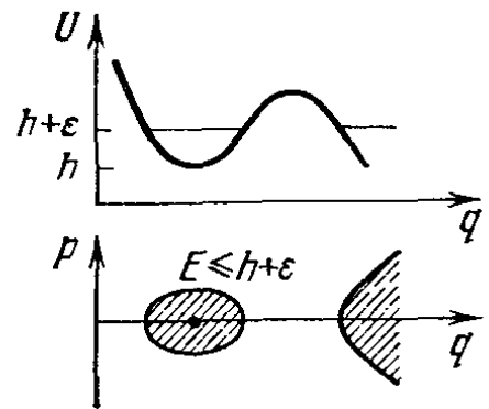
Рис. 75. Устойчивое положение равновесия
