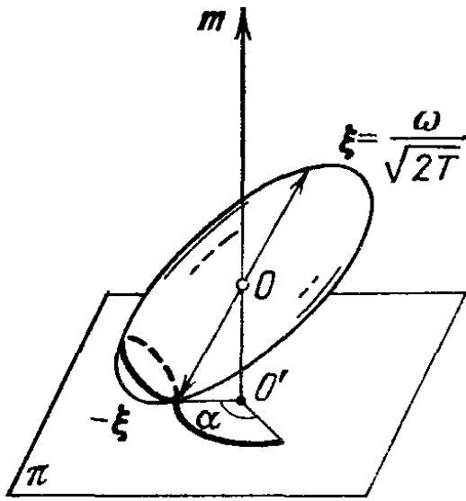
Рис. 122. Качение эллипсоида инерции по неподвижной плоскости
