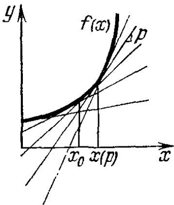
Рис. 45. Инволютивность преобразования Лежандра
