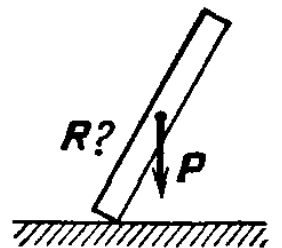
Рис. 74. Сила реакции стола
