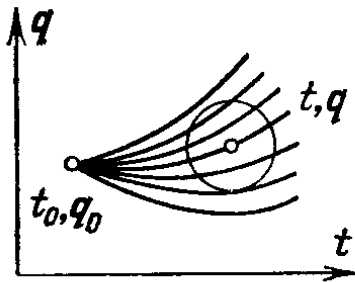
Рис. 198. Центральное поле экстремалей
