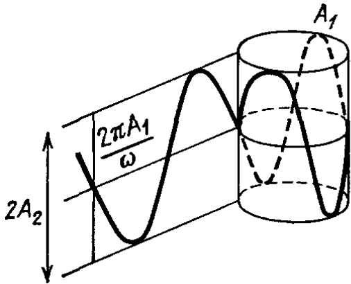
Рис. 19. Построение фигуры Лиссажу
