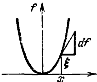
Рис. 140. Дифференциал функции
