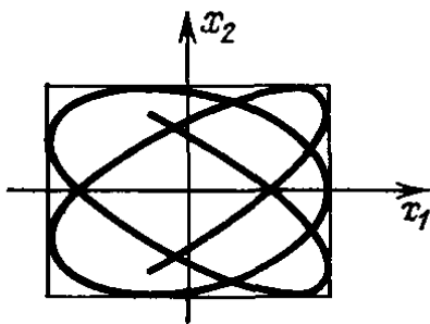
Рис. 21. Фигура Лиссажу с \omega \approx 1
