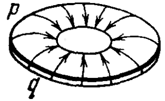
Рис. 173. Локально гамильтоново поле на торе
