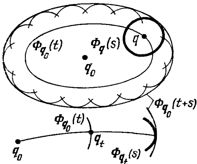
Рис. 193. Огибающая волновых фронтов
