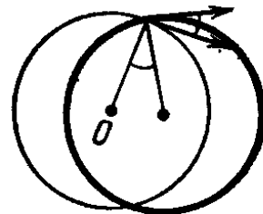
Рис. 36. Орбита, близкая к круговой
