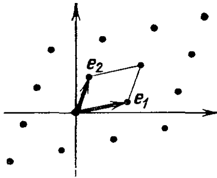
Рис. 214. Дискретная подгруппа плоскости
