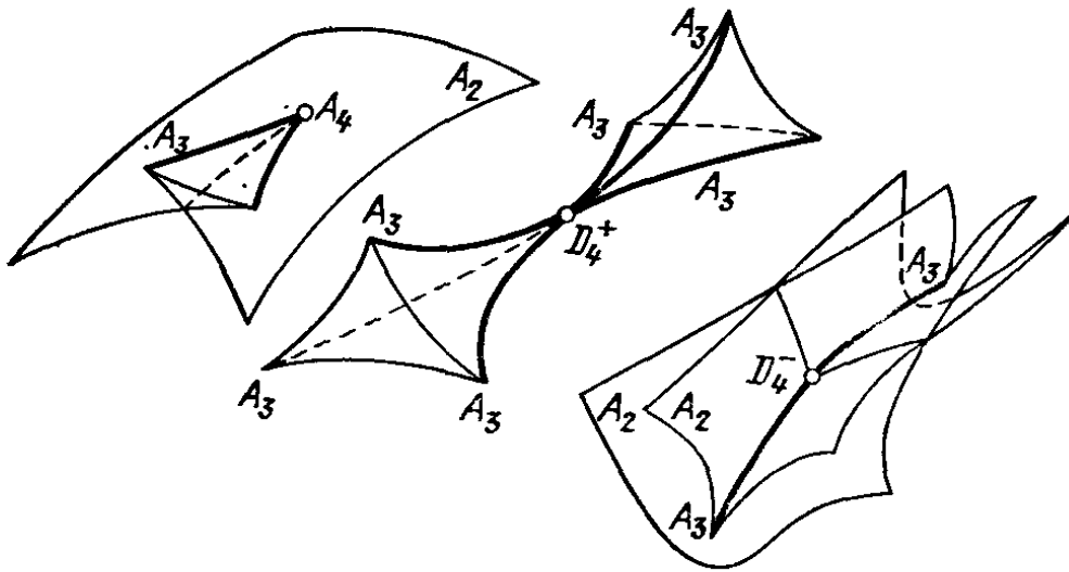
Рис. 246. Типичные особенности каустик в трехмерном пространстве
