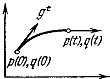
Рис. 47. Фазовый поток
