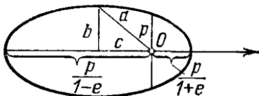
Рис. 35. Кеплеров эллипс
