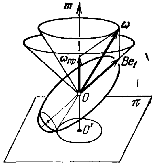
Рис. 124. Качение эллипсоида вращения по неподвижной плоскости
