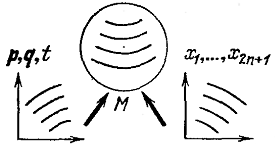
Рис. 184. Замена переменных в уравнениях Гамильтона
