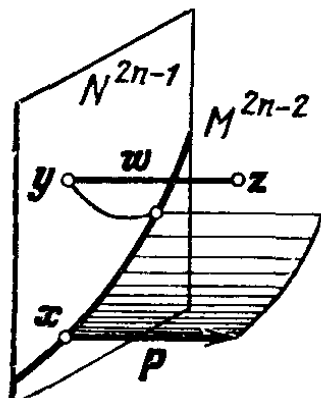
Рис. 179. Построение симплектических координат
