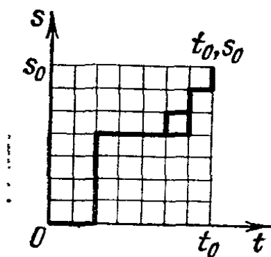
Рис. 170. К доказательству коммутативности потоков
