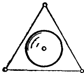
Рис. 117. Эллипсоид инерции равностороннего треугольника
