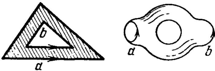
Рис. 165. Гомологичные циклы
