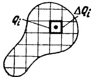
Рис. 118. Сплошное твердое тело
