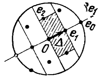
Рис. 215. К доказательству леммы о дискретных подгруппах
