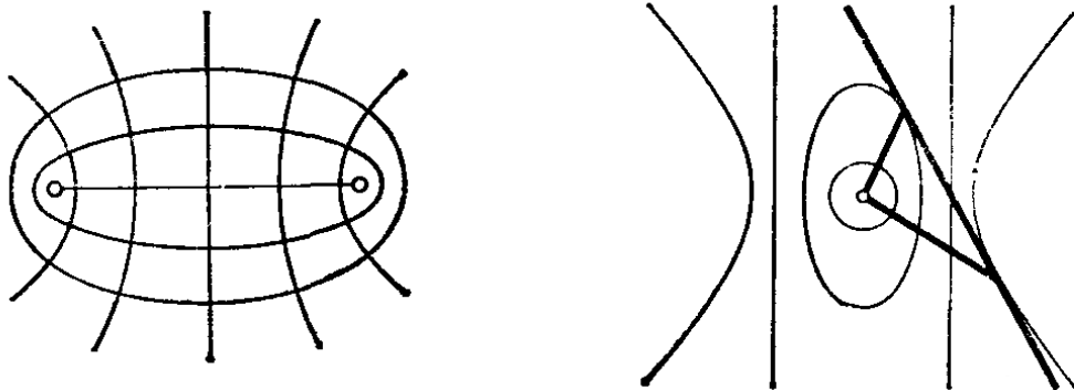
Рис. 248. Конфокальное семейство и евклидов пучок
