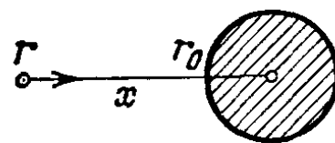
Рис. 7. Поле тяготения Земли
