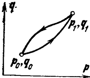
Рис. 185. Замкнутость формы p dq - P dQ
