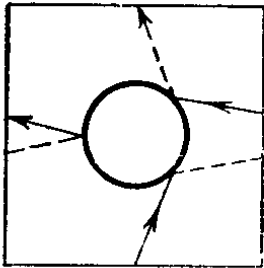
Рис. 235. Торический бильярд с рассеивающей круглой стенкой
