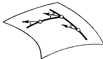
Рис. 230. Параллельное перенесение вдоль геодезической ломаной
