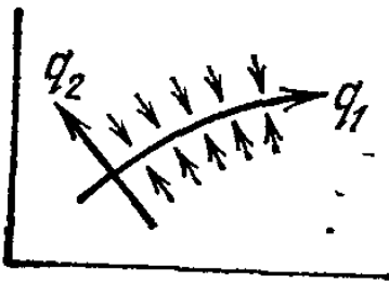
Рис. 54. Связь как бесконечно сильное поле
