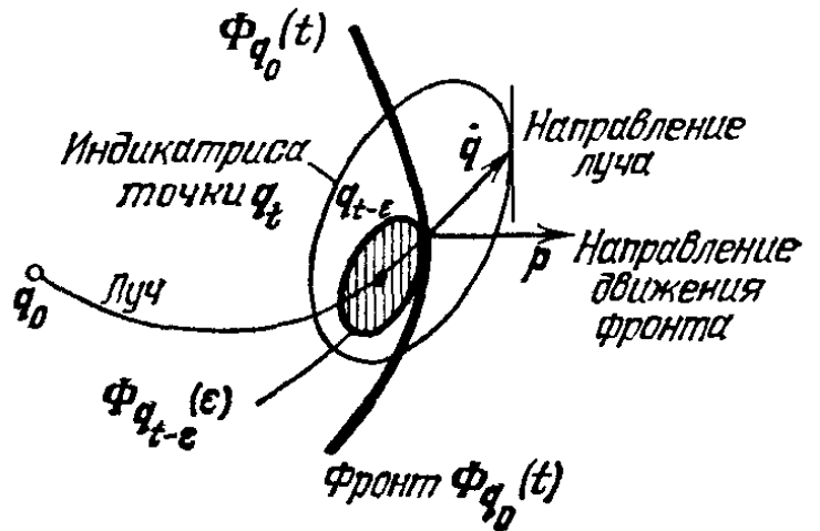
Рис. 197. Сопряженность направлений луча и фронта
