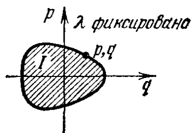
Рис. 228. Адиабатический инвариант, одномерной системы
