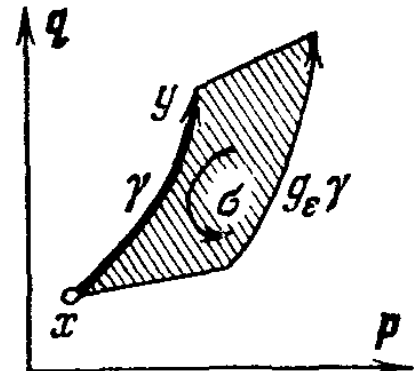
Рис. 210. Геометрический смысл функции Гамильтона
