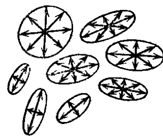
Рис. 192. Неизотропная неоднородная среда
