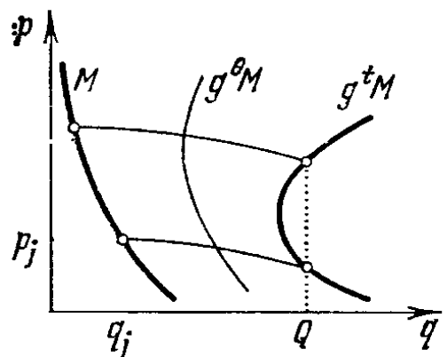
Рис. 244. Преобразование лагранжевых многообразий фазовым потоком
