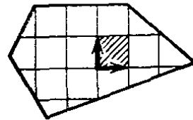
Рис. 148. Интегрирование k -формы в k -мерном пространстве
