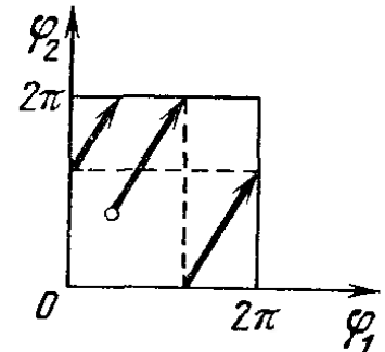
Рис. 221. Условно-периодическое движение
