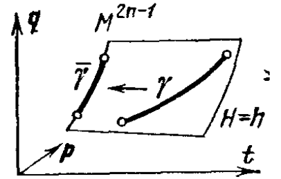
Рис. 186. Понижение порядка гамильтоновой системы
