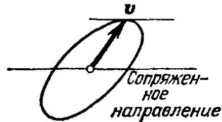
Рис. 196. Сопряженная гиперплоскость
