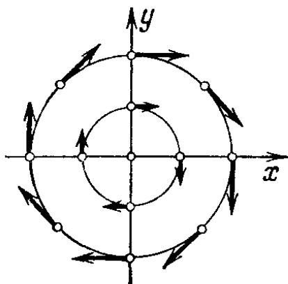
Рис. 9. Фазовая плоскость уравнения \ddot{x} = -x
