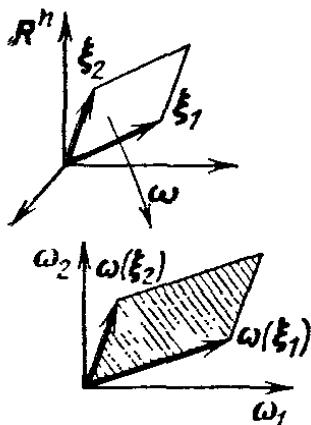
Рис. 139. Определение внешнего произведения двух 1-форм
