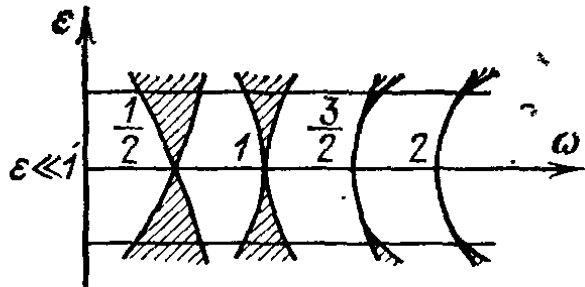
Рис. 99. Зоны параметрического резонанса
