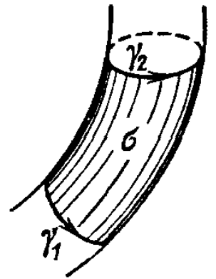
Рис. 180. Трубка ротора
