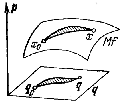
Рис. 219. Независимость интеграла p dq на M_f от пути
